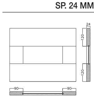
cestone frassino bianco assoluto (opz.2460) absolute white ash deep drawer (code 2460)
