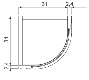
PENSILE TERMINALE stondata con anta END WALL UNIT with curved door
