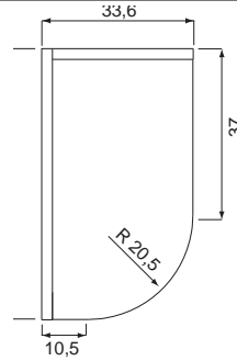
BASE TERMINALE stondata a giorno open END BASE UNIT rounded
