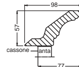
disegno cornice design cornice
