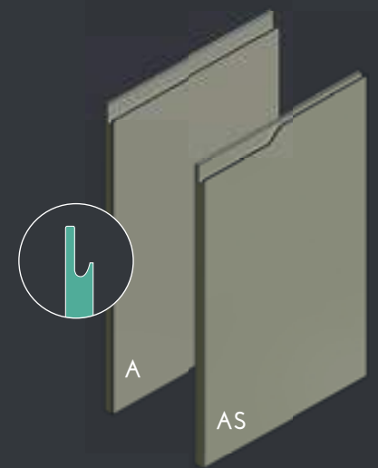
TIPO A - AS ANTE PER BASI CON PRESA ORIZZONTALE CON E SENZA SAGOMATURA
