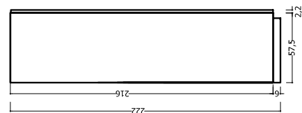
COLONNE FORNO OVEN COLUMNS
