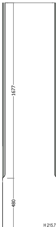
ANTA COLONNA ATTREZZATA COLUMN EQUIPPED DOOR
