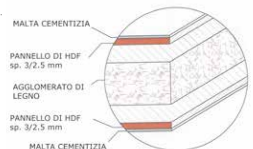
sezione anta door section
