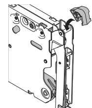
SCHEMA MONTAGGIO LIMITATORE PER RIBALTA H 48 FLAP DOOR LIMITER INSTALLATION DIAGRAM H 48
